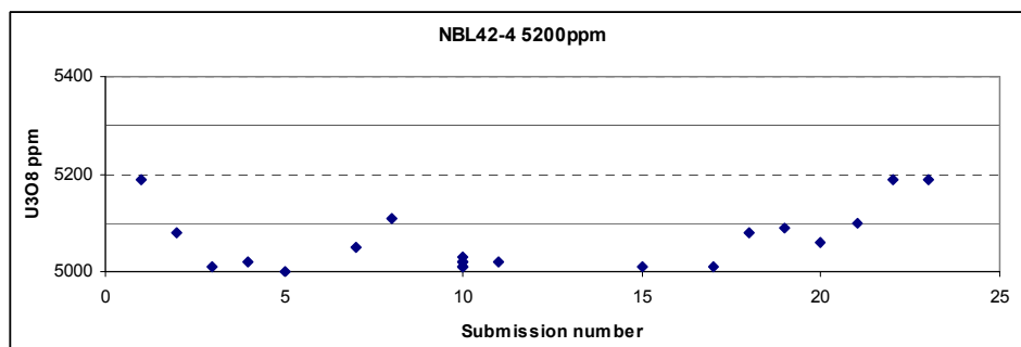
Figure 33: Assays of reference standard NBL42-4 ALS laboratory
